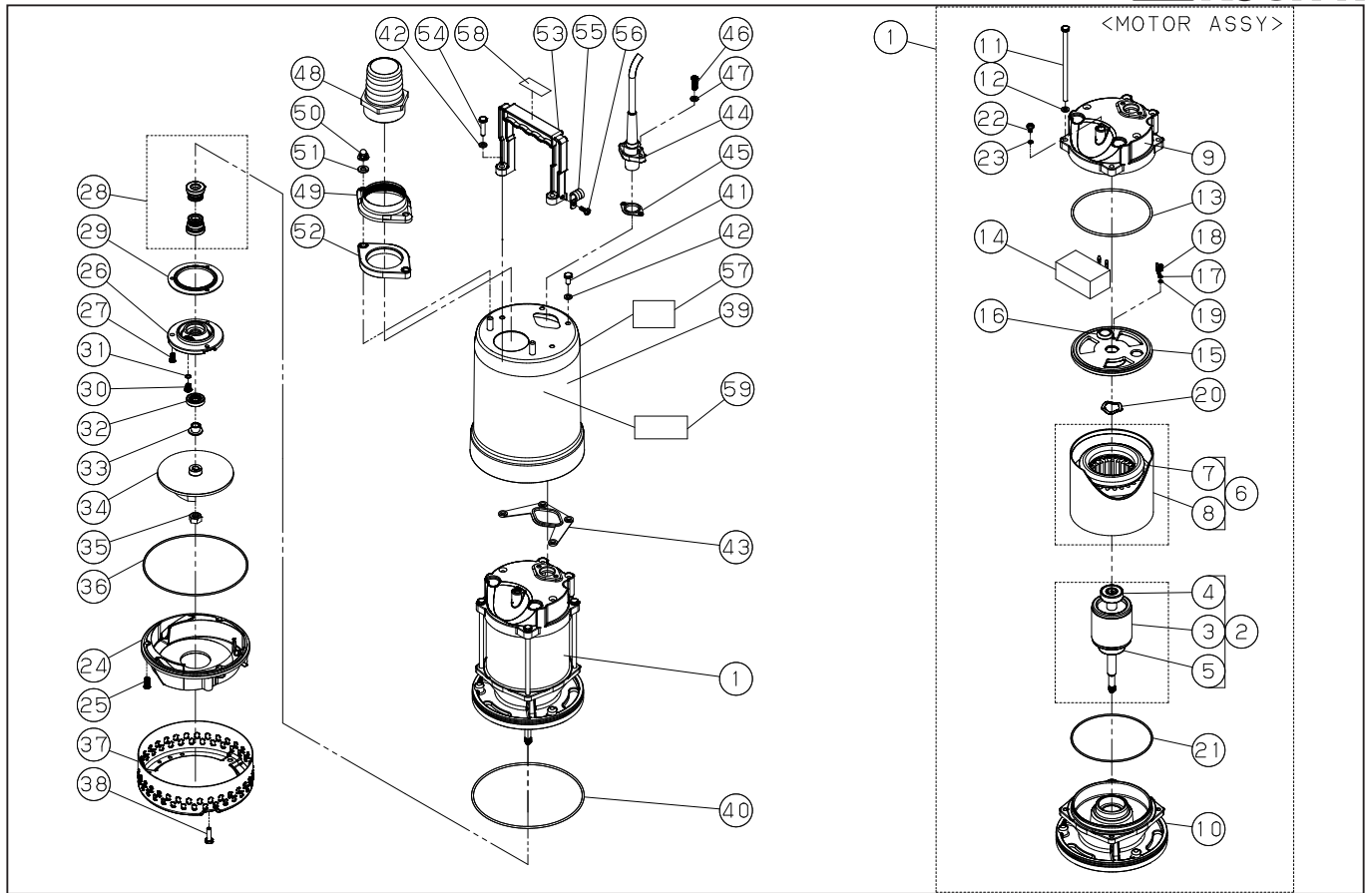
DWG No.077850301 MODELE : PXJ-400 FORM : PXJ-400-BAB-0
